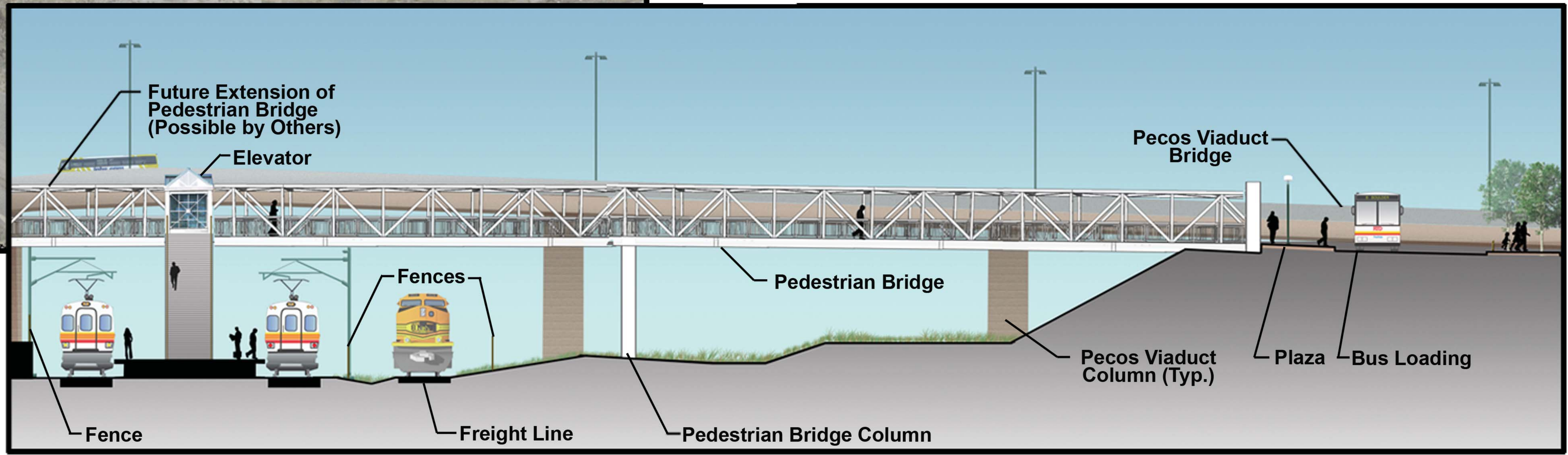
Section A-A
