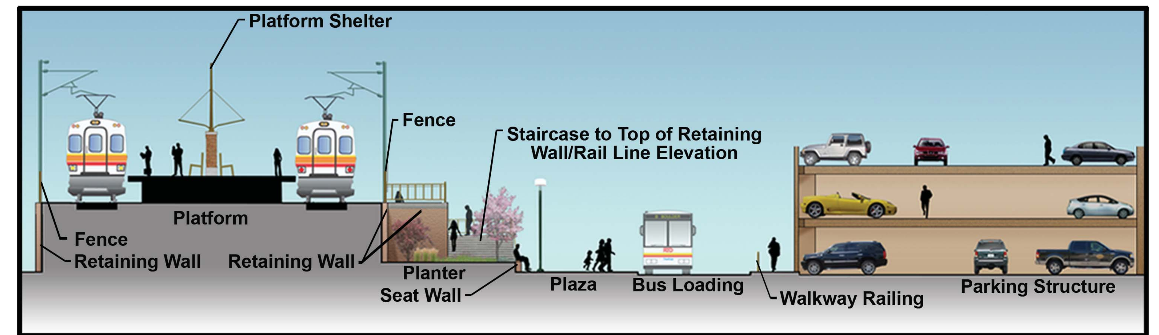
Section D-D
