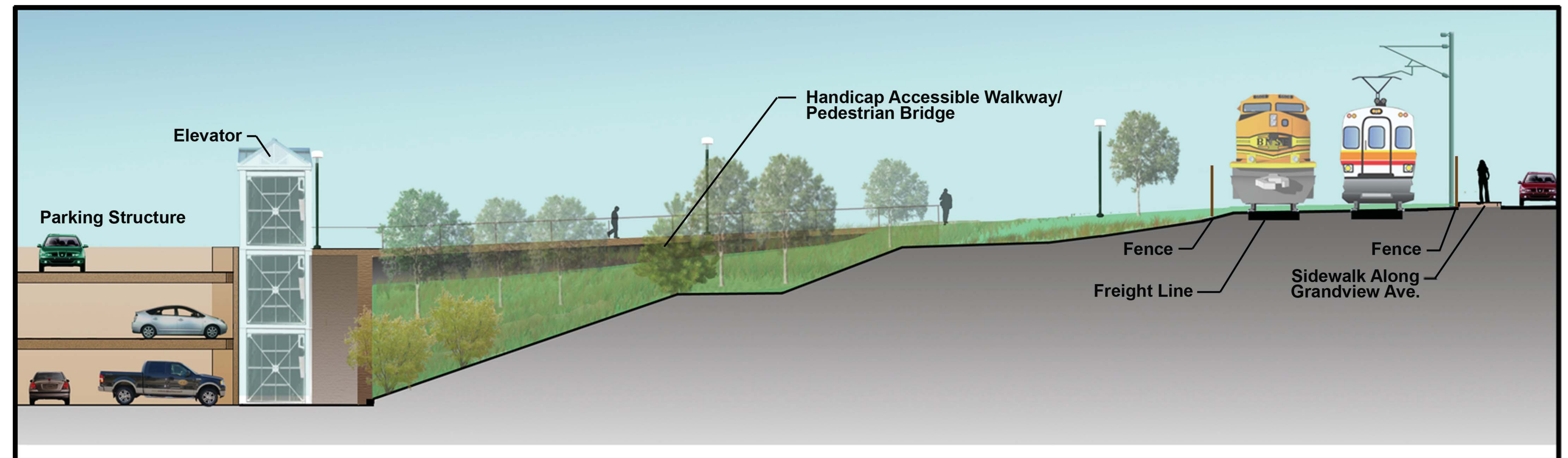
Section D-D
